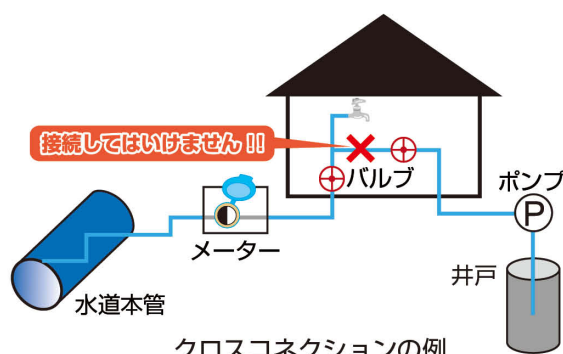
クロスコネクションの例
